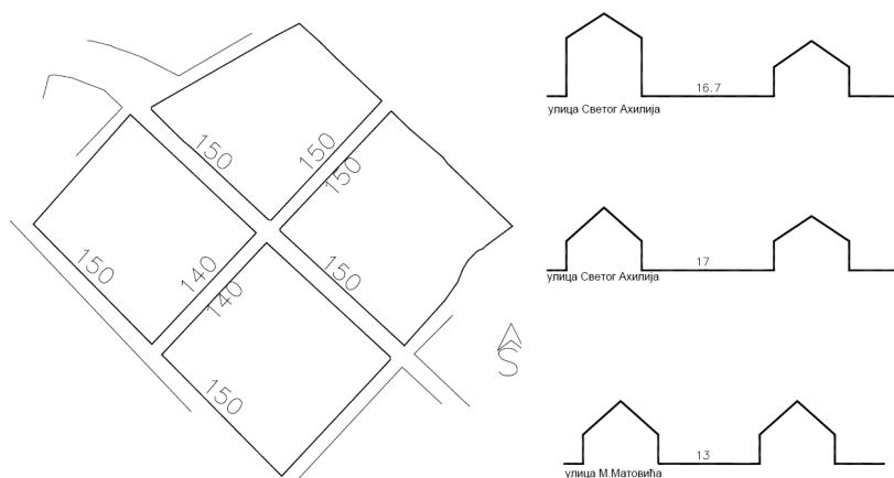
Слика 08. Ариље, улична мрежа, пресек кроз главну и попречну улицу
